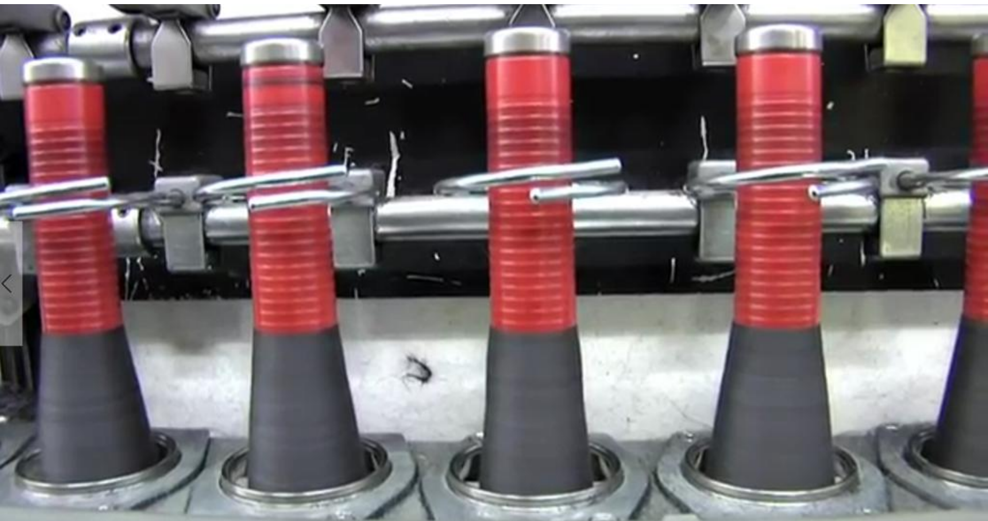
příze na potáčích – prstencový dopřádací stroj
