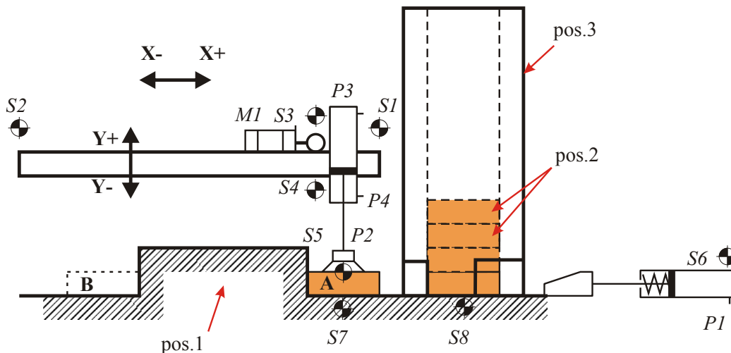
Obrázek 1: Situační schéma manipulátoru
