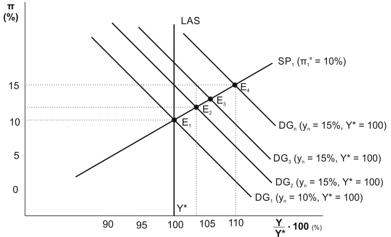
Obr. 4 Přizpůsobovací cesta – neměnná míra očekávané inflace
