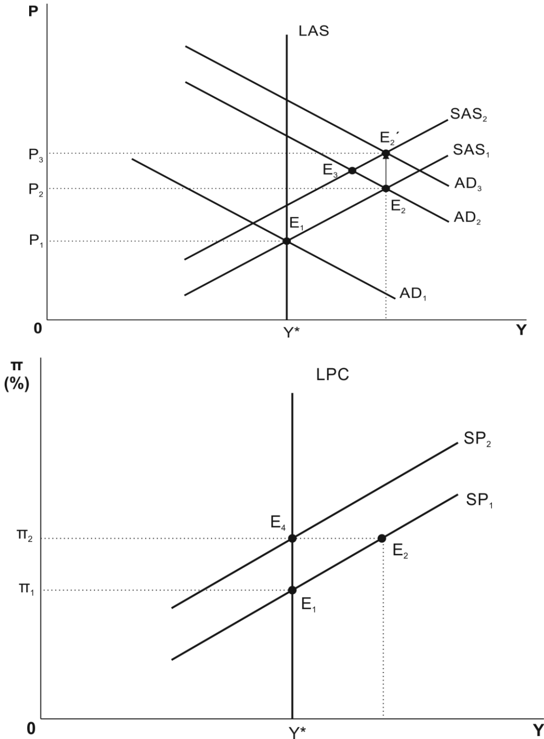
Obr. 1 Odvození křivky SP
