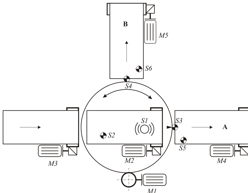
Obrázek 1: Situační schéma otočné stanice na dopravníkové trati
