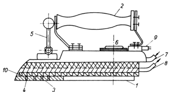
Obr. 67 Funkční schéma žehličky
