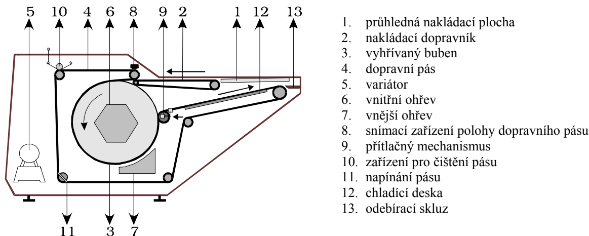
Obr. 70 Bubnový podlepovací stroj (nakládání i odběr oděvních součástí na stejném místě)
