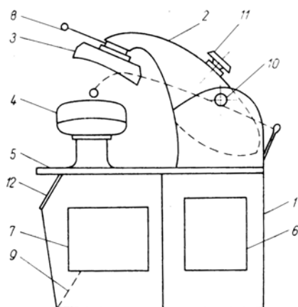
Obr. 68 Funkční schéma žehličního stroje základního provedení
